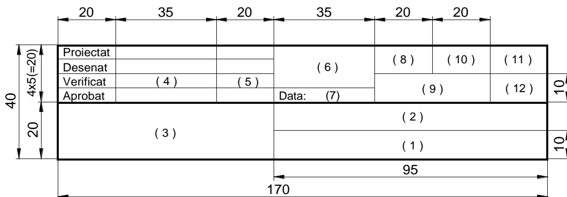
Fig. 3.6. Exemplu de compartimentare a indicatorului desenului tehnic (Cioat, V. G., Desen tehnic industrial. Elemente teoretice și aplicații , Ed. PIM, Iași, 2010)
