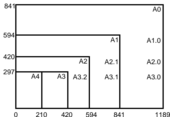
Fig. 3.5. Formate alungite utilizate în desenul tehnic (Cioat, V. G., Desen tehnic industrial. Elemente teoretice și aplicații , Ed. PIM, Iași, 2010)
