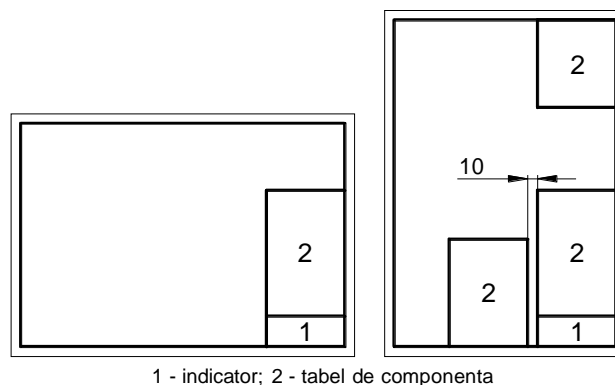
Fig. 3.9. Poziționarea tabelului de componen
