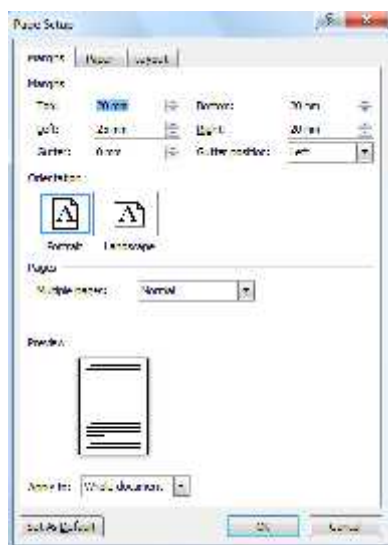
Fig.3.1. Setarea paginii
