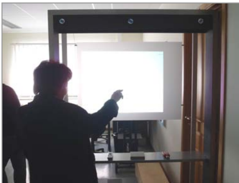
Testare bază de date și accesare resurse pedagogice „Portal Interactiv BRIS și interfață touchless 3D”. Utilizator - Carmen Inge ALIC, Universitatea Politehnica din Timișoara
